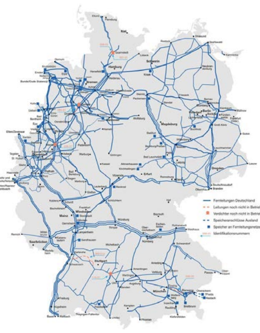
Abbildung 61: Höchstspannungsnetz [VDE] und Gas-Fernleitungsnetz [Fern].
