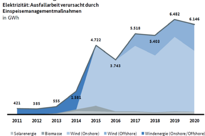
Abbildung 22: Abgeregelter elektrische Energie [BNA2].
