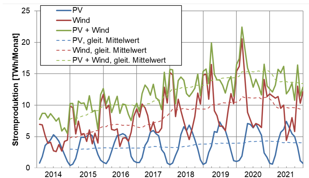
Abbildung 25: Monatssummen PV- und Windstromproduktion, Daten aus [ISE4].
