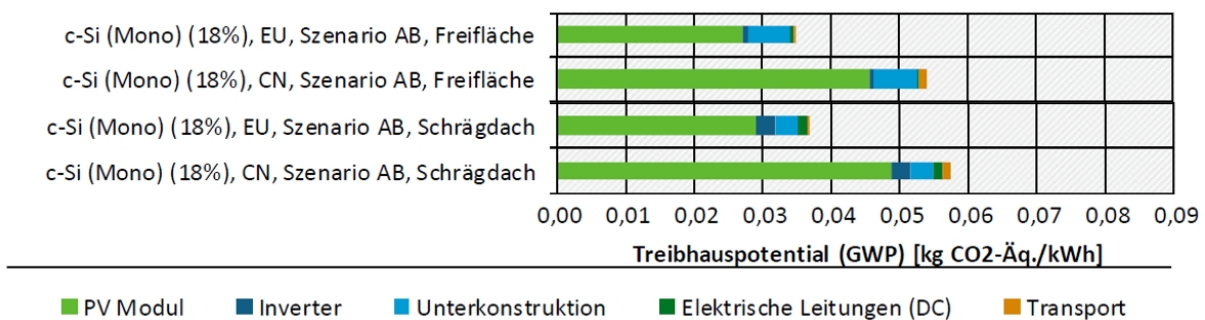
Abbildung 43: Treibhauspotential der Stromerzeugung mit mono c-Si PV für Dach- und Freiflächenanlagen [UBA7].
