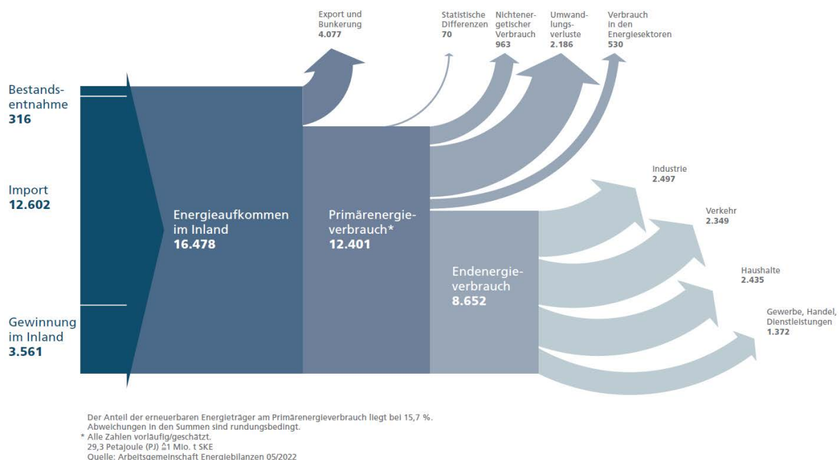
Abbildung 47: Energieflussbild 2021 für Deutschland, Angaben in Petajoule [AGEB2].
