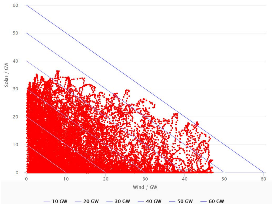
Abbildung 24: Mittlere Leistung für die Einspeisung von Sonnen- und Windstrom im Jahr 2021, 15-Minuten-Werte [ISE4].
