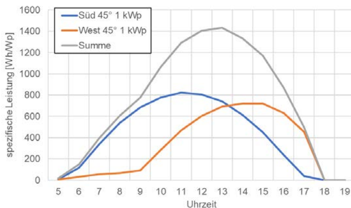
Abbildung 37: Stundenprofil der Stromproduktion an einem klaren Apriltag für verschiedene Dachausrichtungen bei 45° Dachneigung, unverschattet, Standort Freiburg, berechnet online mit https://re.jrc.ec.europa.eu/pvg_tools/en/ .
